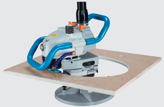
GPW510A & GPW510B'i beraber kullanarak İç Kenar Frezeleme işleminin uygulanması
